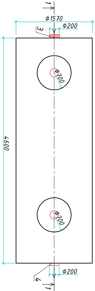
Вид сверху
