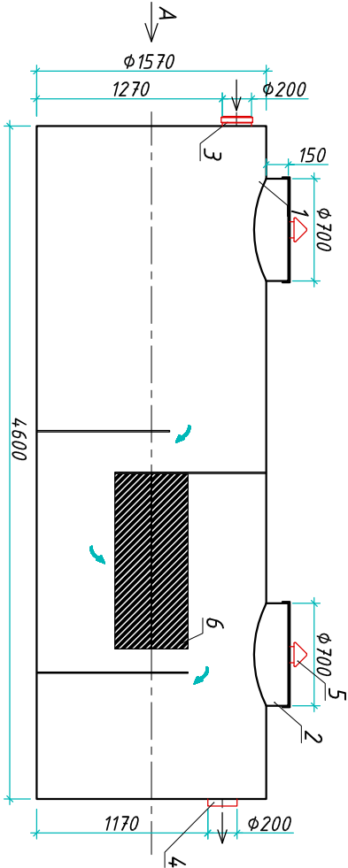
Разрез 1-1
