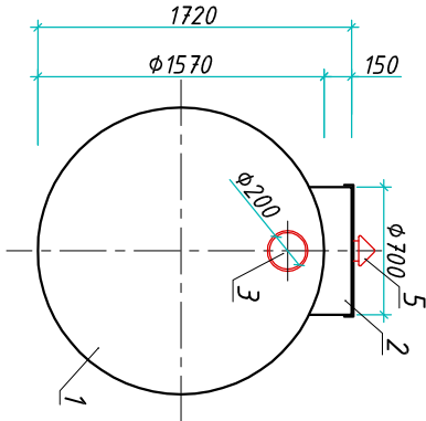
Вид А
